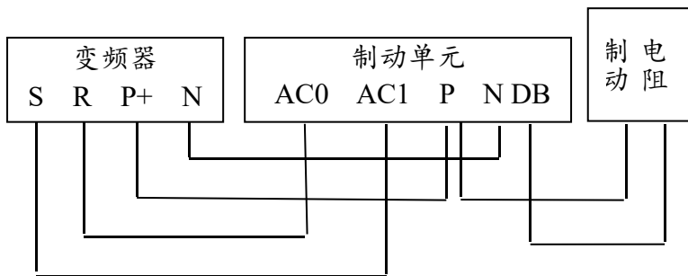
22kW 以上制动单元接线图
