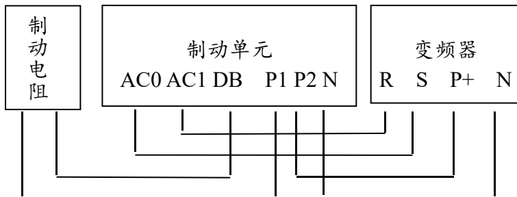
SZ10G11/22 制动单元接线图
